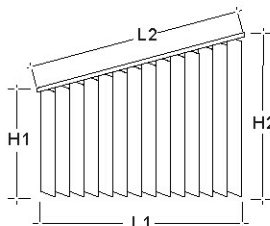
FIS Inclínada Superior
